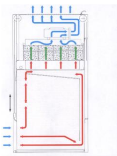
Die Luftführung
